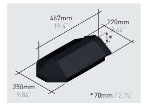
Q122*K | Angular hip / end ridge klinker
