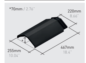
Q120*K | Angular ridge klinker
