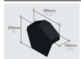
Q124*K | Angular end cap klinker
